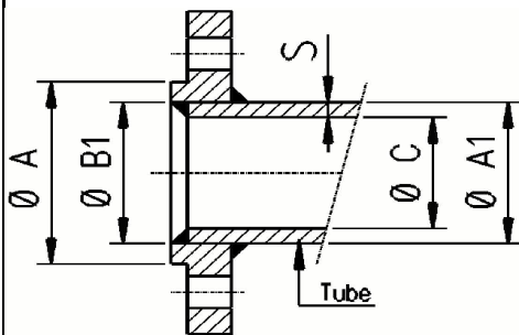
FLANGE TYPE 01
